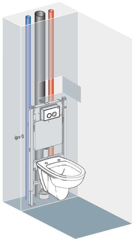
Монтажный элемент Geberit Duofix UP182 для подвесного унитаза Арт. 458.160.00.1
