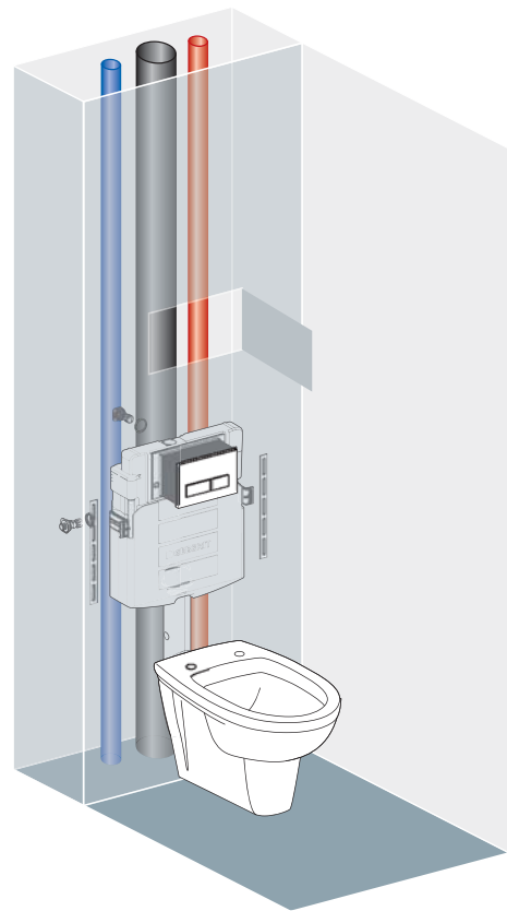
Встраиваемый бачок Geberit UP320 для приставного унитаза Арт. 109.300.00.1
