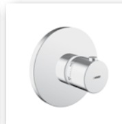
Термостат скр. монтажа 4866 9501 хромированный, без блокировки, плюс 4000 0000 *базовый блок скр. монтажа
