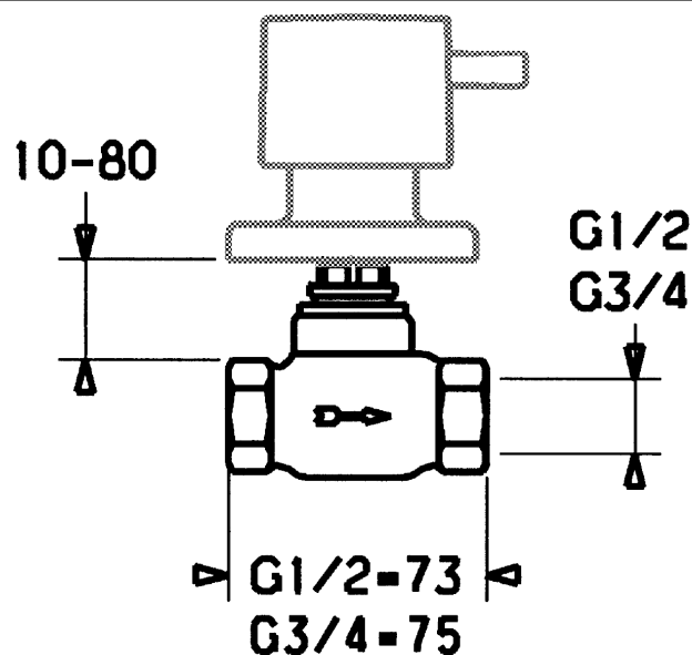
Produktzeichnung
