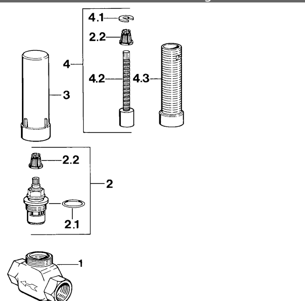
Produktzeichnung
