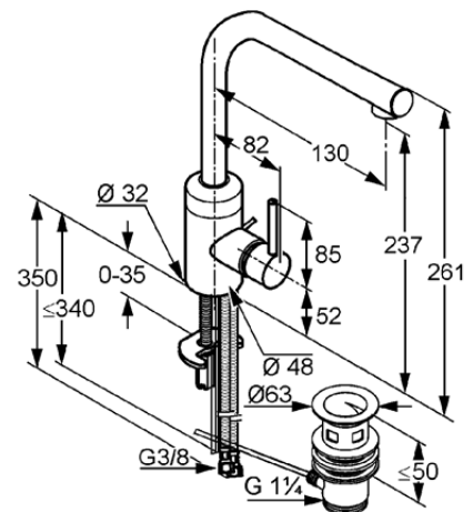
РАЗМЕРЫ
