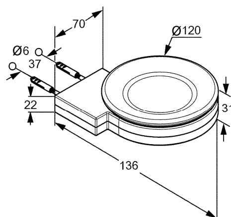
Размеры
