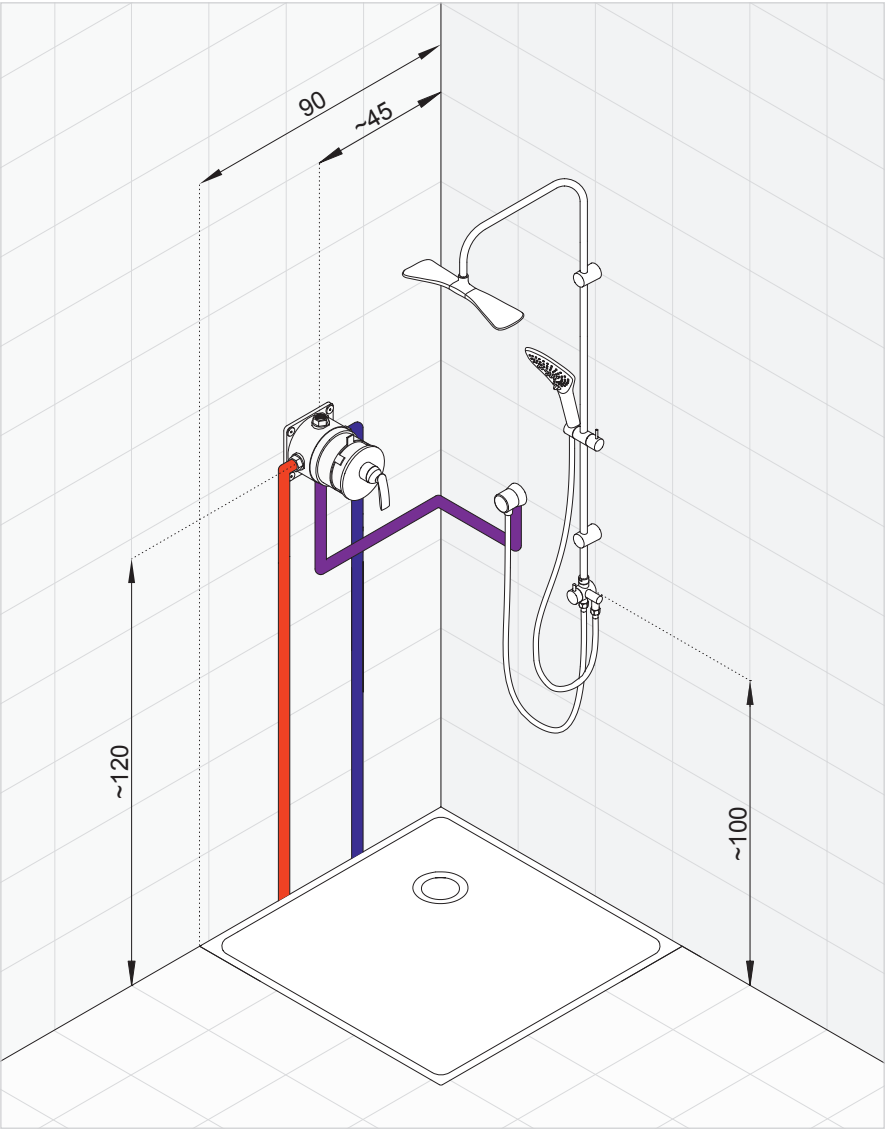
Гарнитур KLUDI DUAL SHOWER SYSTEM имеет два источника воды, регулируемые интегрированным переключателем. Смешанная вода подается через соединение для шланга.
